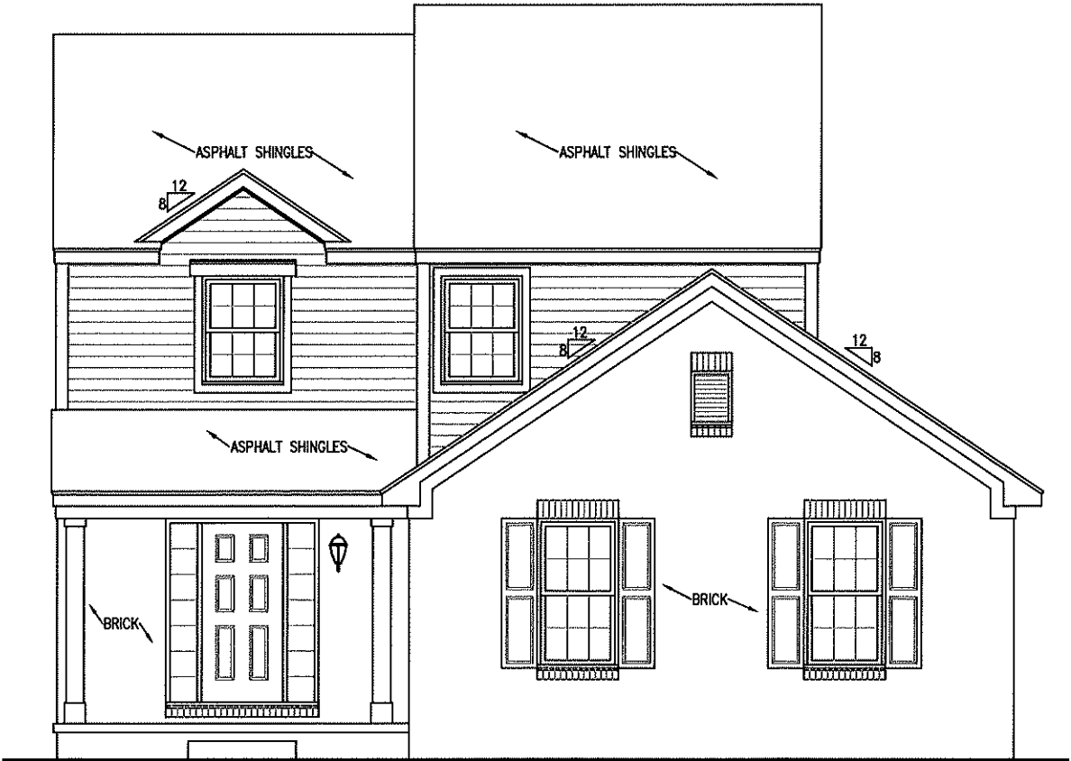
ELEVATION - B
